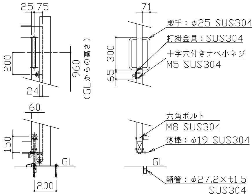
詳細図 S = 1 / 20
