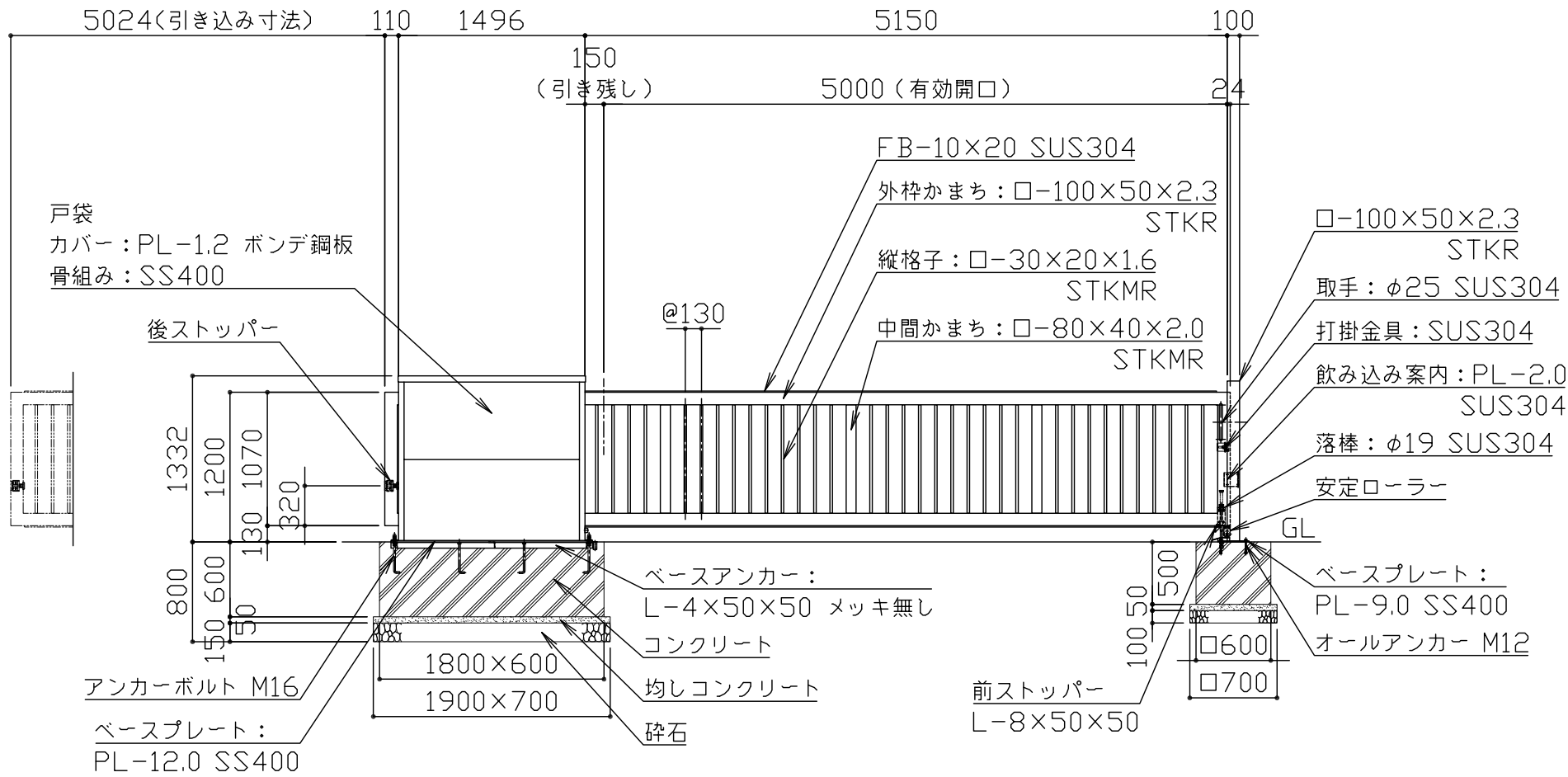
立面図 S = 1 / 50
