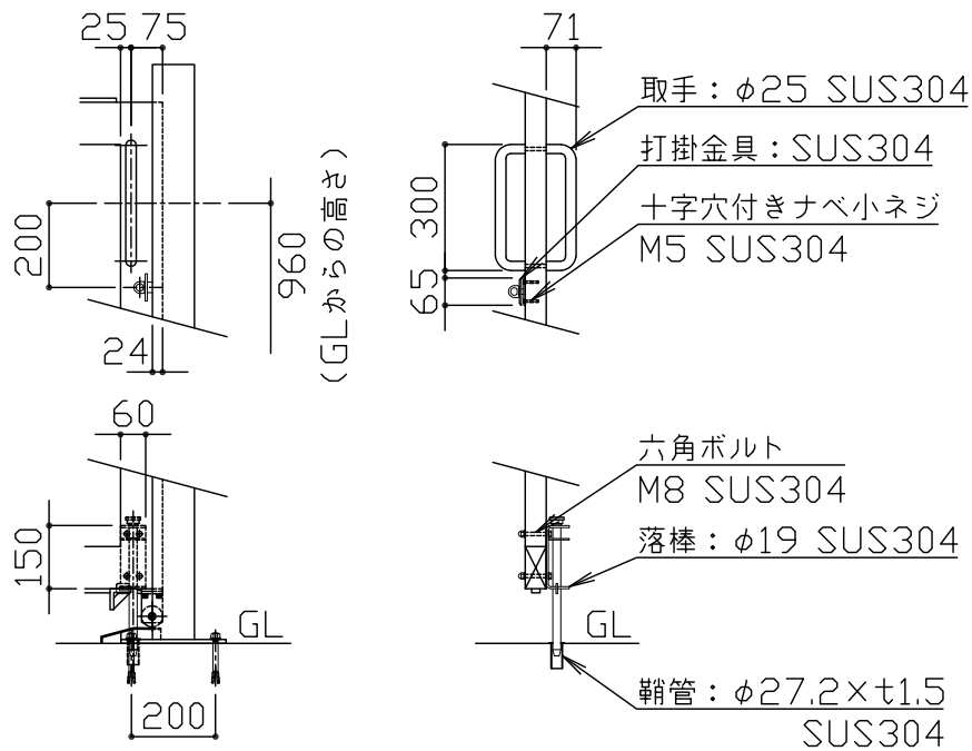
詳細図 S = 1 / 20
