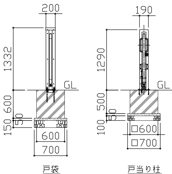
側面図 S = 1 / 50
