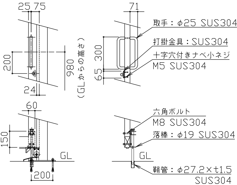
詳細図 S = 1 / 20
