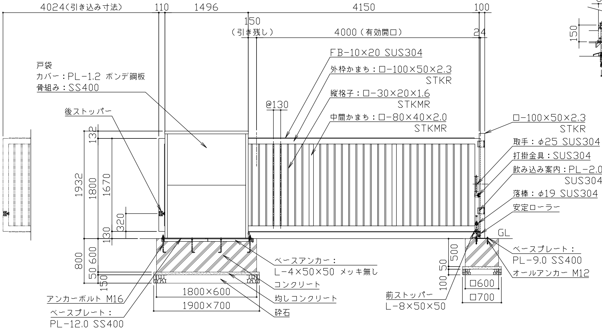
立面図 S = 1 / 40
