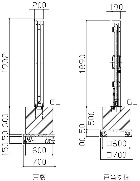
側面図 S = 1 / 40
