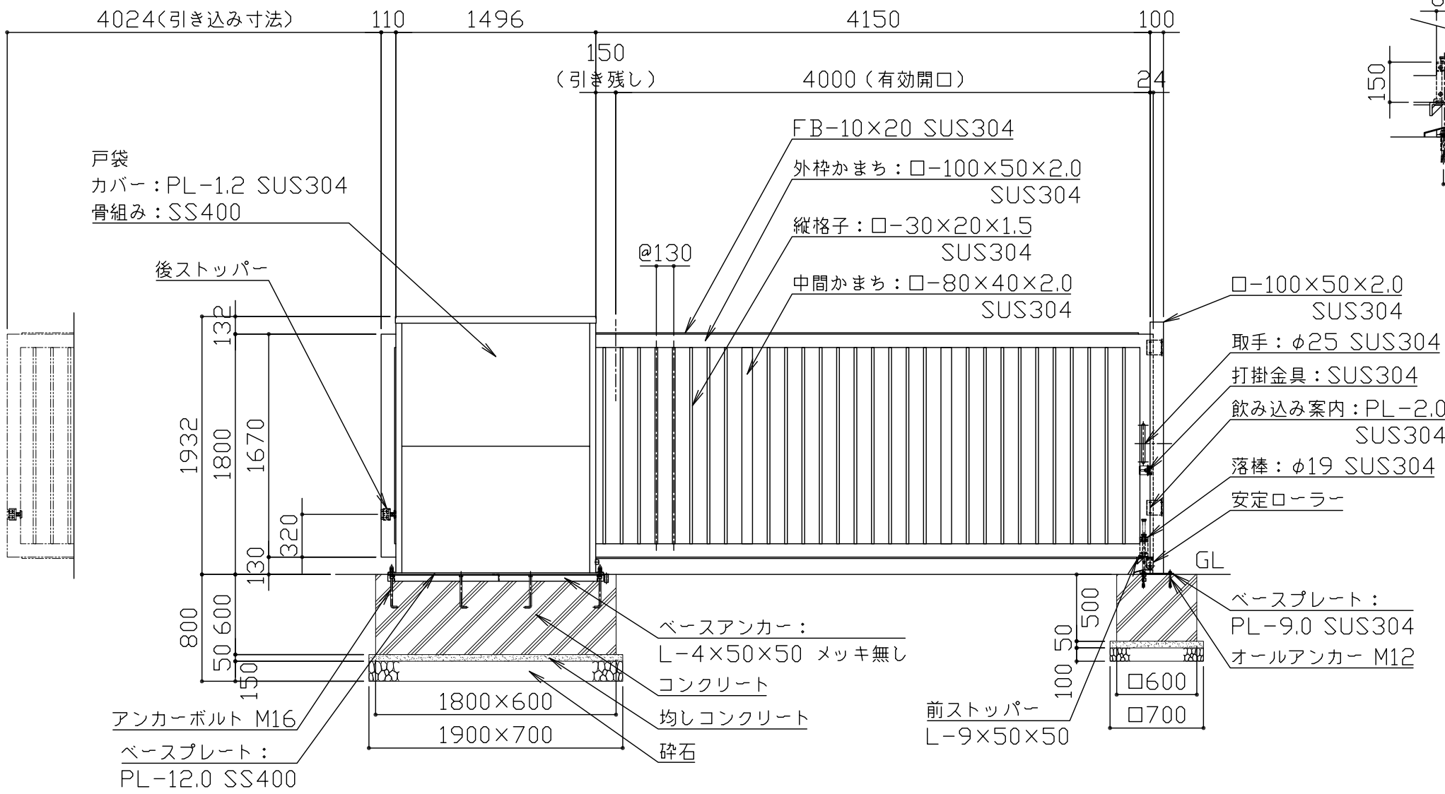
立面図 S = 1 / 40
