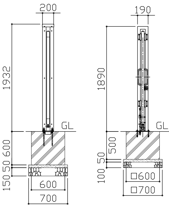
側面図 S = 1 / 40
