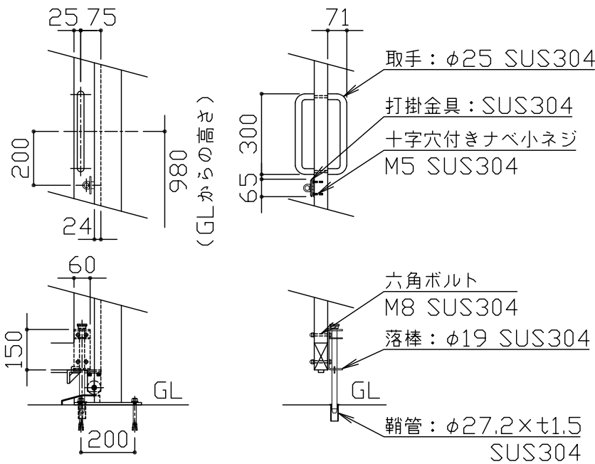
詳細図 S = 1 / 20
