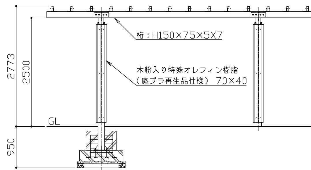
立面图 S = 1/50
