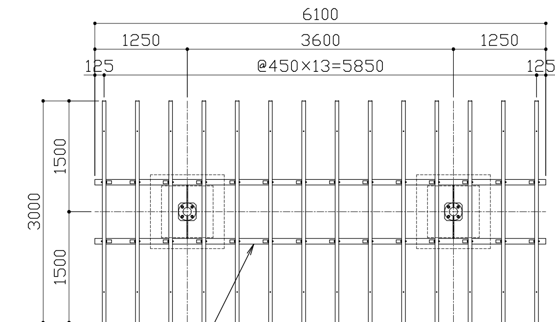
桁：H150×75×5×7
