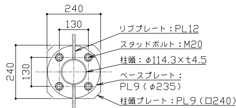
柱頭部 S = 1 / 10
