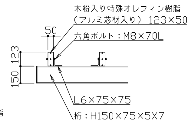
栈木取付部 S = 1/20
