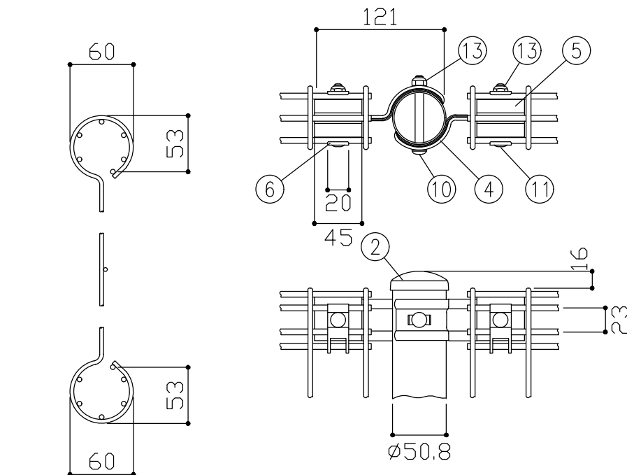
A部詳細図 S = 1 / 5
