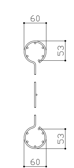
本体パネル詳細図 S = 1 / 5
