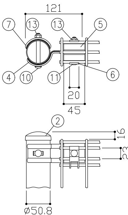
C部詳細図 S = 1 / 5
