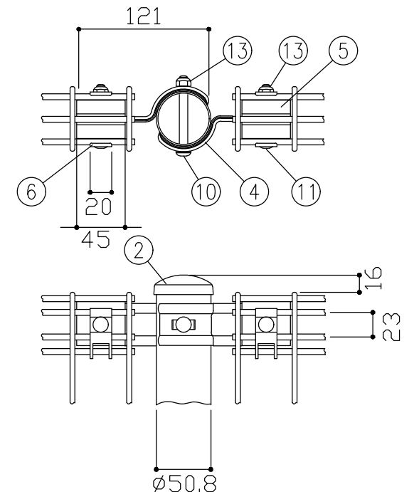
A部詳細図 S = 1 / 5
