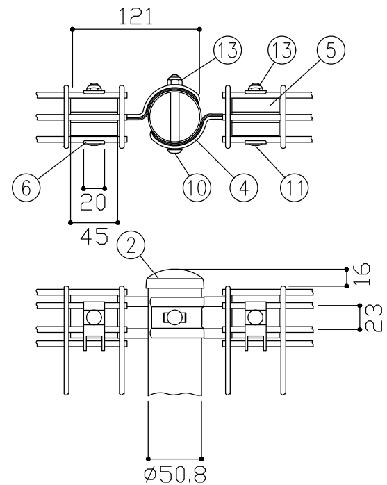
A部詳細図 S = 1 / 5
