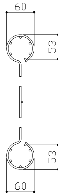
本体パネル詳細図 S = 1 / 5
