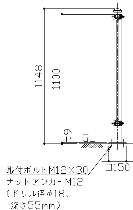
側面図 S = 1 / 2 0
