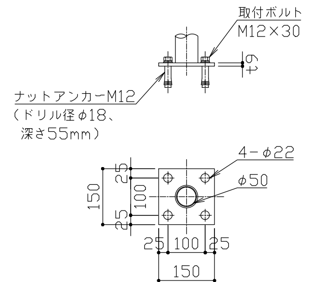
ベースプレート詳細図 S = 1 / 1 0
