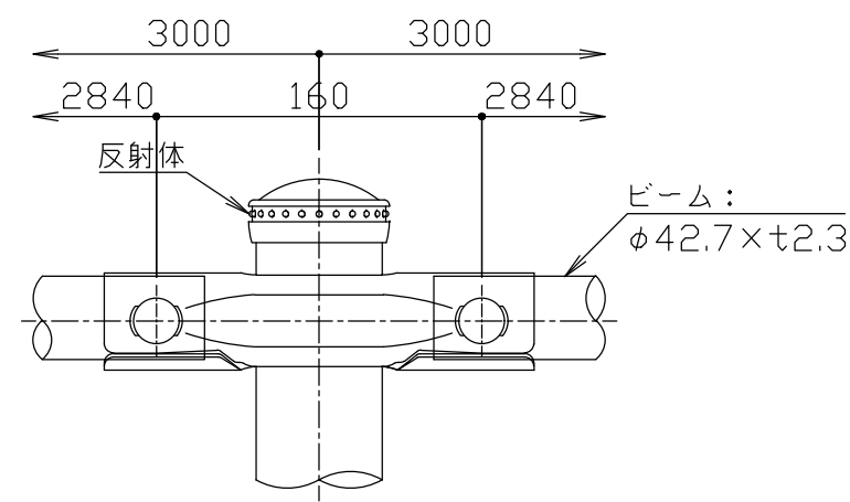
立面図 S = 1 / 2 0
