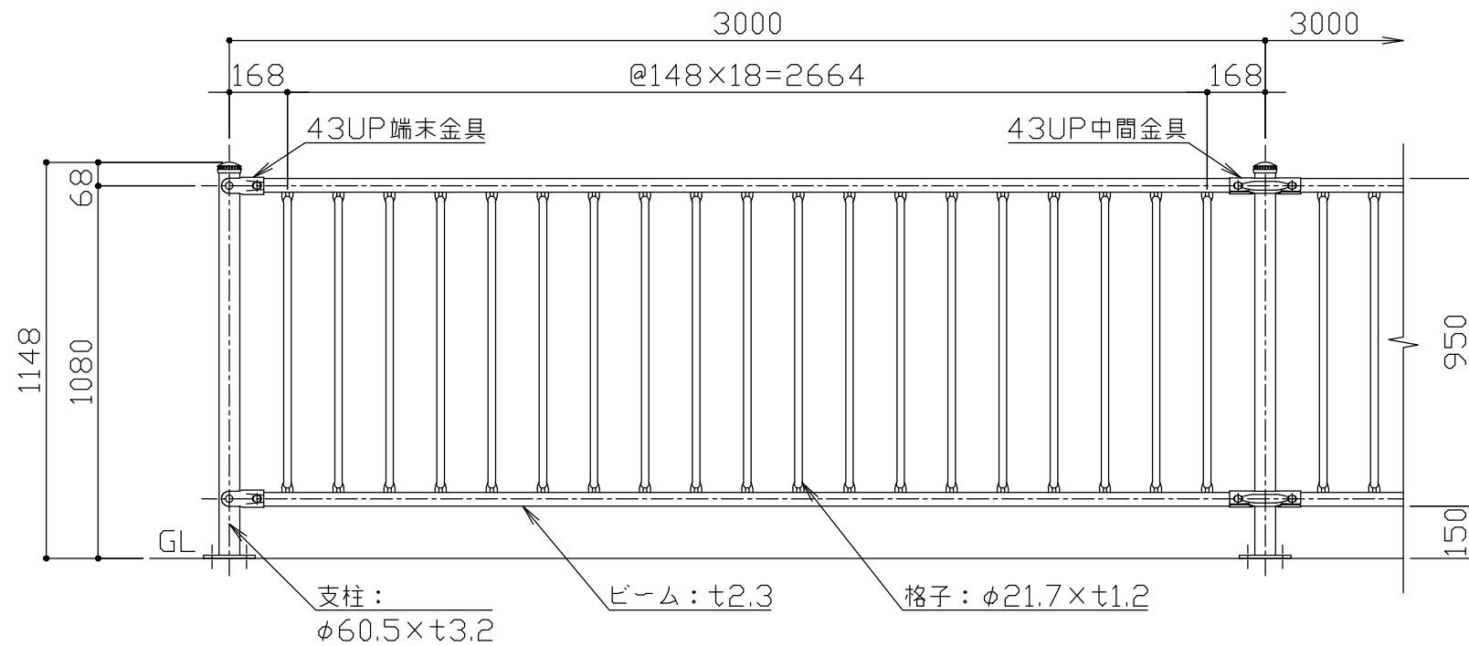
立面図 S = 1 / 2 0
