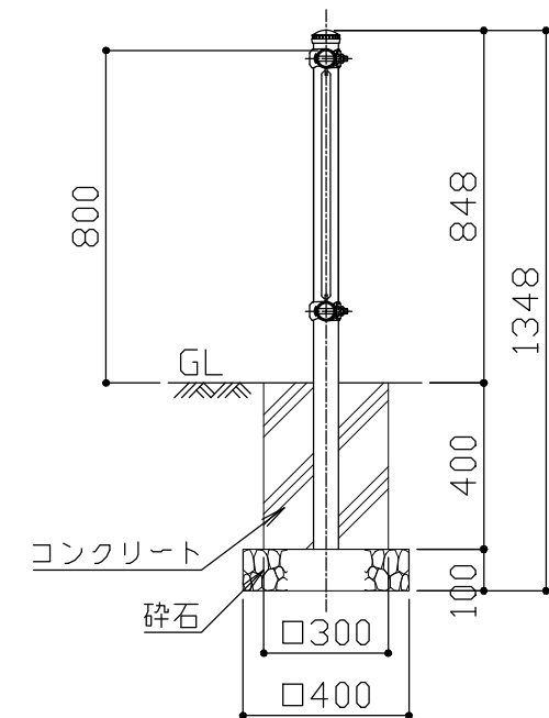
側面図 S = 1 / 20
