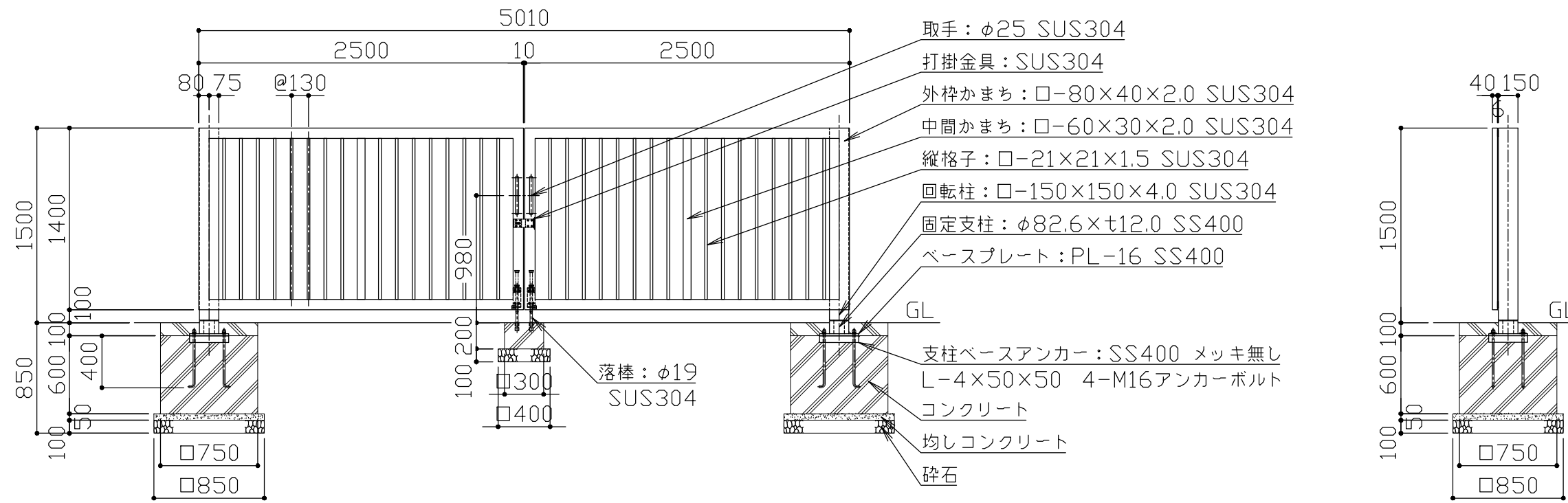
立面図 S = 1 / 40
