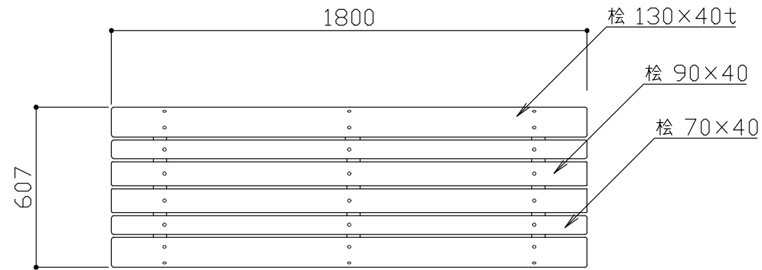
平面図 S = 1 / 20
