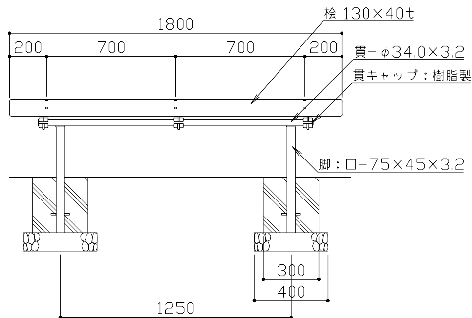
立面図 S = 1 / 20
